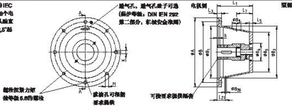
钟形罩 (A型结构VDMA 24561标准)
